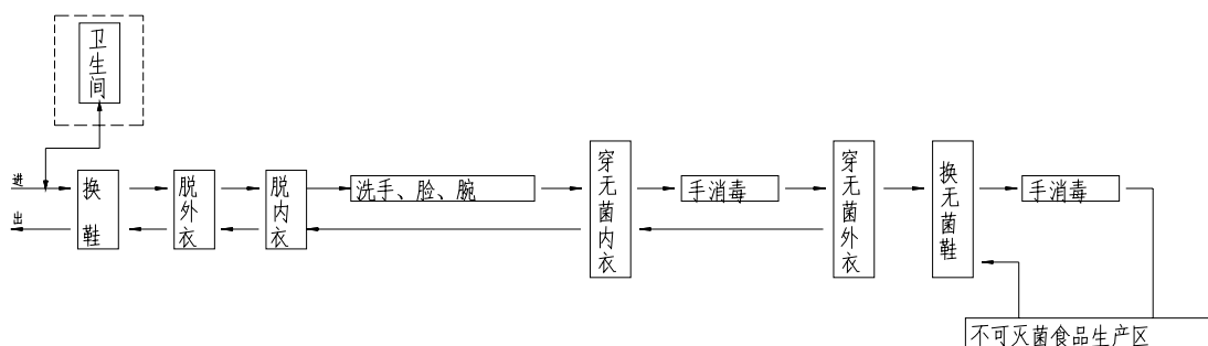
图 5.4.4 不可灭菌食品生产区人员净化程序
