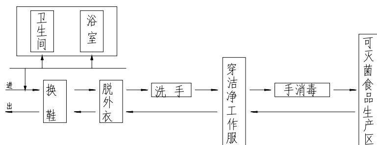
图 5.4.3 可灭菌食品生产区人员净化程序
